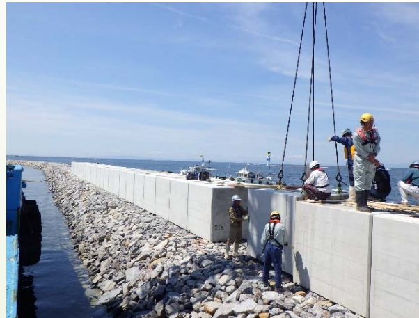
名古屋港湾事務所 護岸工事整備状況（全景）
